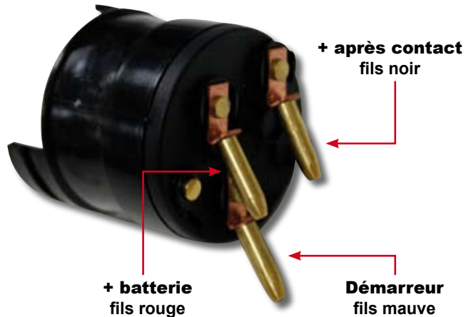
Branchements Contacteur Mehari réf. : 1005020
