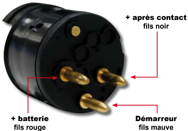
Branchements Contacteur 2CV réf. : 3005020
